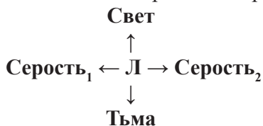
Рис. 1. Аксиологические аттракторы
