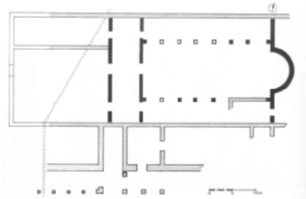
План на базилика №2 в Диоклецианопол (Маджаров 1993, 175, изоб.135)
