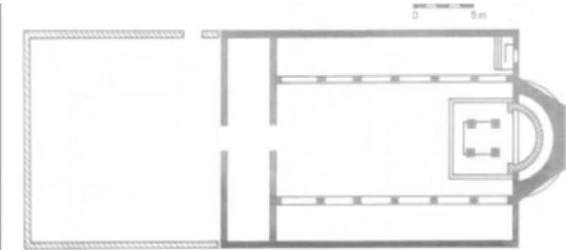
План на базилика №3 в Диоклецианопол (Маджаров 1993, 177, изоб.136)
