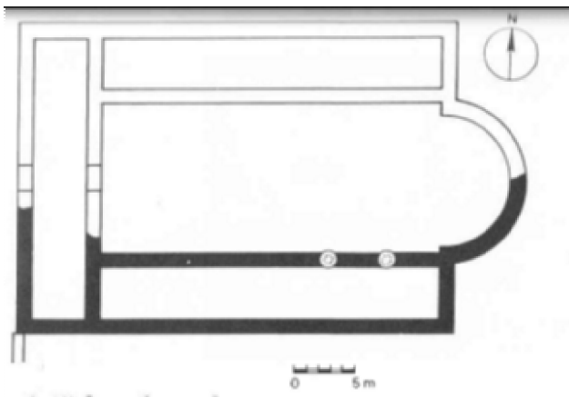
План на базилика № 5 в Диоклецианопол (Маджаров 1993, 179, изоб. 144)
