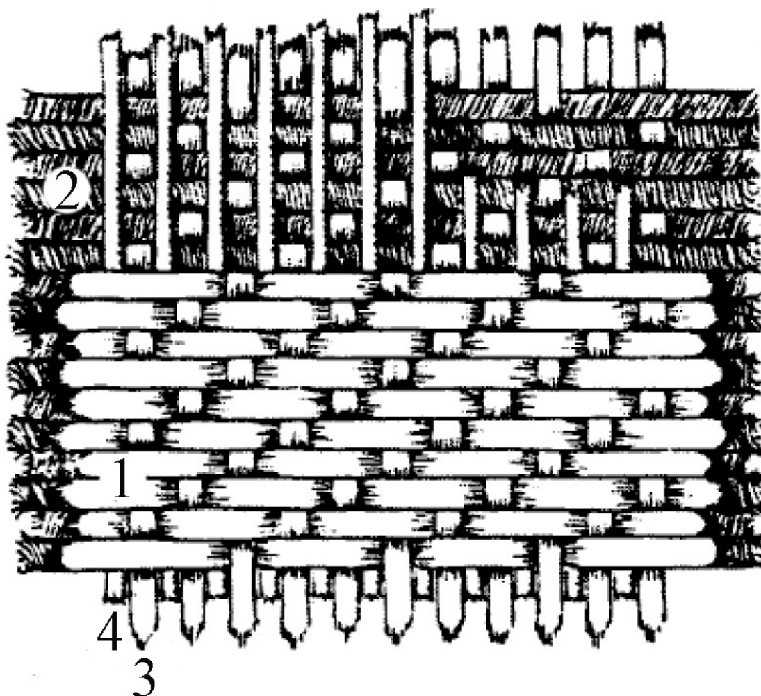
Обр. 4. Схема на вътъчнолицев сложен кепър – самит: 1 – лицев вътък; 2 – вътък, изграждащ гърба; 3 – преплитаща основа; 4 – свободна основа (по М. Фехнер)
